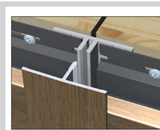
Alu H-Profil (zweiteilig)
