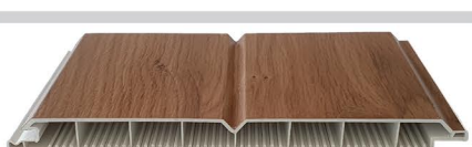
Hohlkammerprofil 040 verstärktes Profil mit V-Fuge Deckbreite 200 mm
