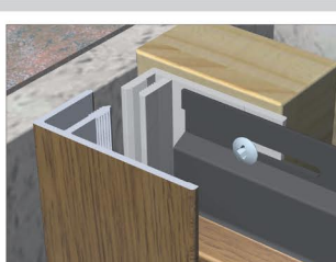
Alu U-Profil (zweiteilig)
