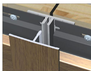
Alu H-Profil (zweiteilig)
